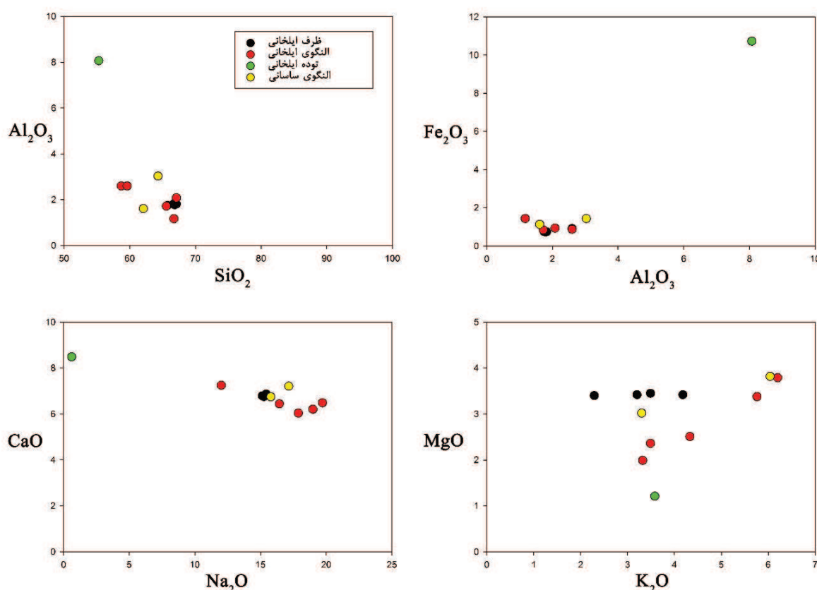
شکل ۲- نمودارهای نسبت SiO_2 در برابر Al_2O_3 ، Al_2O_3 در برابر Fe_2O_3 ، Na_2O در برابر CaO و K_2O در برابر MgO در نمونه‌های شیشه محوطه ارزانفود. شباهت ترکیب شیمیایی در نمونه‌ها (به جز نمونه توده شیشه‌ای، AF-13) و به خصوص در چهار نمونه ظرف دوره ایلخانی به خوبی قابل مشاهده است.
