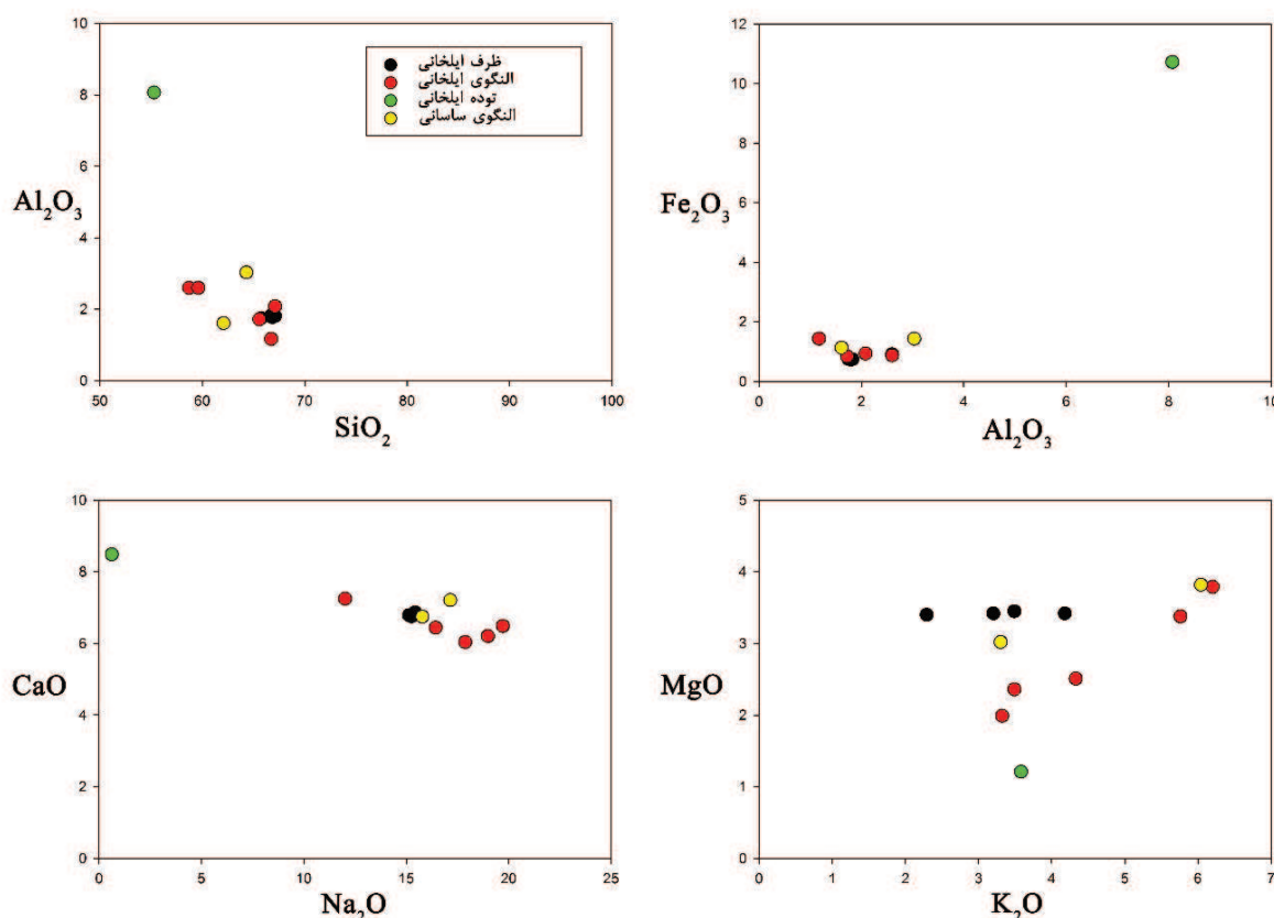
شکل ۲- نمودارهای نسبت SiO_2 در برابر Al_2O_3 ، Al_2O_3 در برابر Fe_2O_3 ، Na_2O در برابر CaO و K_2O در برابر MgO در نمونه‌های شیشه محوطه ارزانفود. شباهت ترکیب شیمیایی در نمونه‌ها (به جز نمونه توده شیشه‌ای، AF-13) و به خصوص در چهار نمونه ظرف دوره ایلخانی به خوبی قابل مشاهده است.
