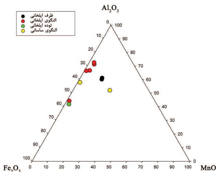
شکل ۳- نمودار سه‌وجهی \text{Fe}_2\text{O}_3 ، \text{Al}_2\text{O}_3 ، \text{MnO} بر اساس نتایج آنالیز نمونه‌های محوطه ارزانفود. نمودار به خوبی نشان می‌دهد که ماده رنگساز اصلی در ترکیب نمونه‌ها آهن است و تفاوت رنگ بین نمونه‌های ظرف و الگو به دلیل حضور میزان بالای \text{MnO} در ترکیب نیست.
