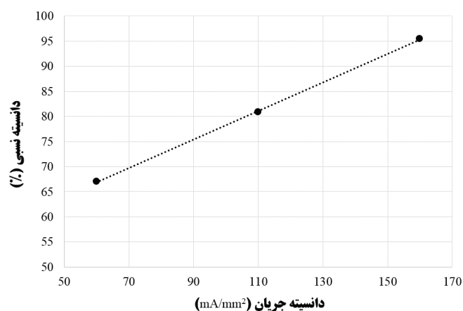
شکل ۷- تاثیر چگالی جریان بر چگالی نمونه‌های سینتر شده تحت شدت میدان 100 \text{ V/cm} در دمای 800^\circ\text{C} با استفاده از خمیر اتصال پلاتین
