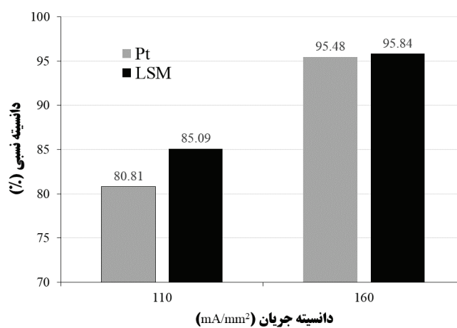
شکل ۸- تاثیر نوع خمیر اتصال بر چگالی نمونه‌های سینتر شده در دمای 800^\circ\text{C} تحت چگالی جریان فلاح مختلف
