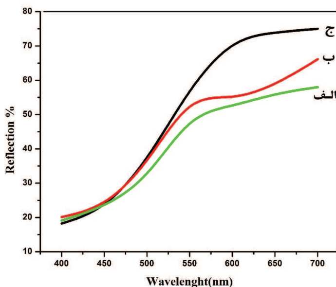
شکل ۴- طیف بازتاب رنگدانه‌های سنتز شده با درصد مختلف دوپه \text{Fe}_2\text{O}_3 (الف) ۰/۰۷ مولار؛ Y1، (ب) ۰/۱۰ مولار؛ Y2 و (ج) ۰/۱۵ مولار؛ Y3
