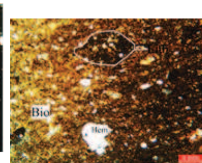
شکل ۶- تصویر میکروسکوپی نمونه ش ۶ سفال خاکستری- سیاه در نور XPL، بزرگنمایی X4
