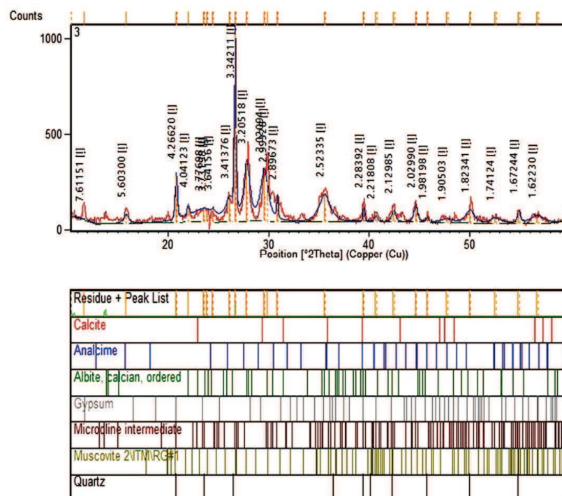
شکل ۵- دیاگرام XRPD قطعه شماره ۳ و فازهای کریستالین شناخته شده
