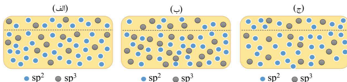
شکل ۴- شماتیک از اثر انرژی یون بر رشد پوشش کربن شبه‌الماس: (الف) E_p > E_{ion} ، نفوذ سطحی غالب است (ب) E_p > E_{ion} ، گونه‌های کربنی به عمق نفوذ می‌کنند و مقدار \text{sp}^3 زیاد می‌شود (ج) E_p \ll E_{ion} ، آسیب ناشی از تصادم شبکه‌ی کربنی رخ می‌دهد و مقدار \text{sp}^2 زیاد می‌شود [۸].
