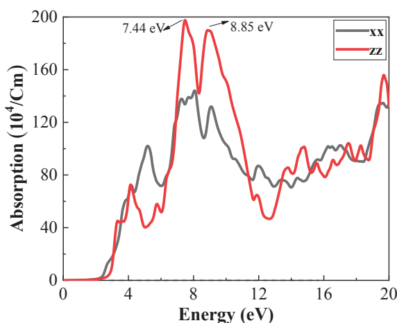
شکل ۹- نمودار ضریب جذب ترکیب ر راستاهای x و z با استفاده از تقریب GGA+U.
