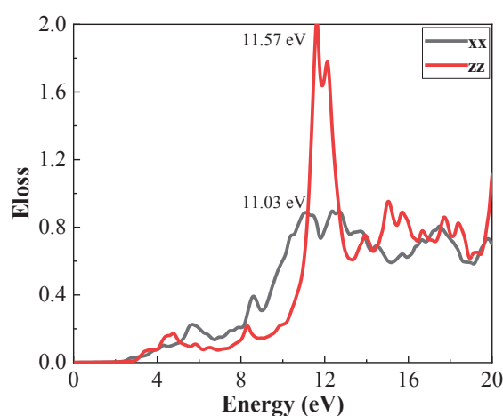
شکل ۸- نمودار تابع اتلاف ترکیب دی‌اکسید تیتانیوم در راستاهای x و z با استفاده از تقریب GGA.
