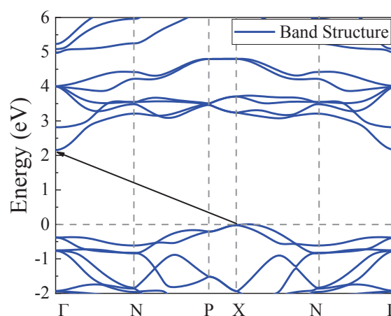
شکل ۴- ساختار نواری ترکیب \text{TiO}_2 با استفاده از تقریب GGA
