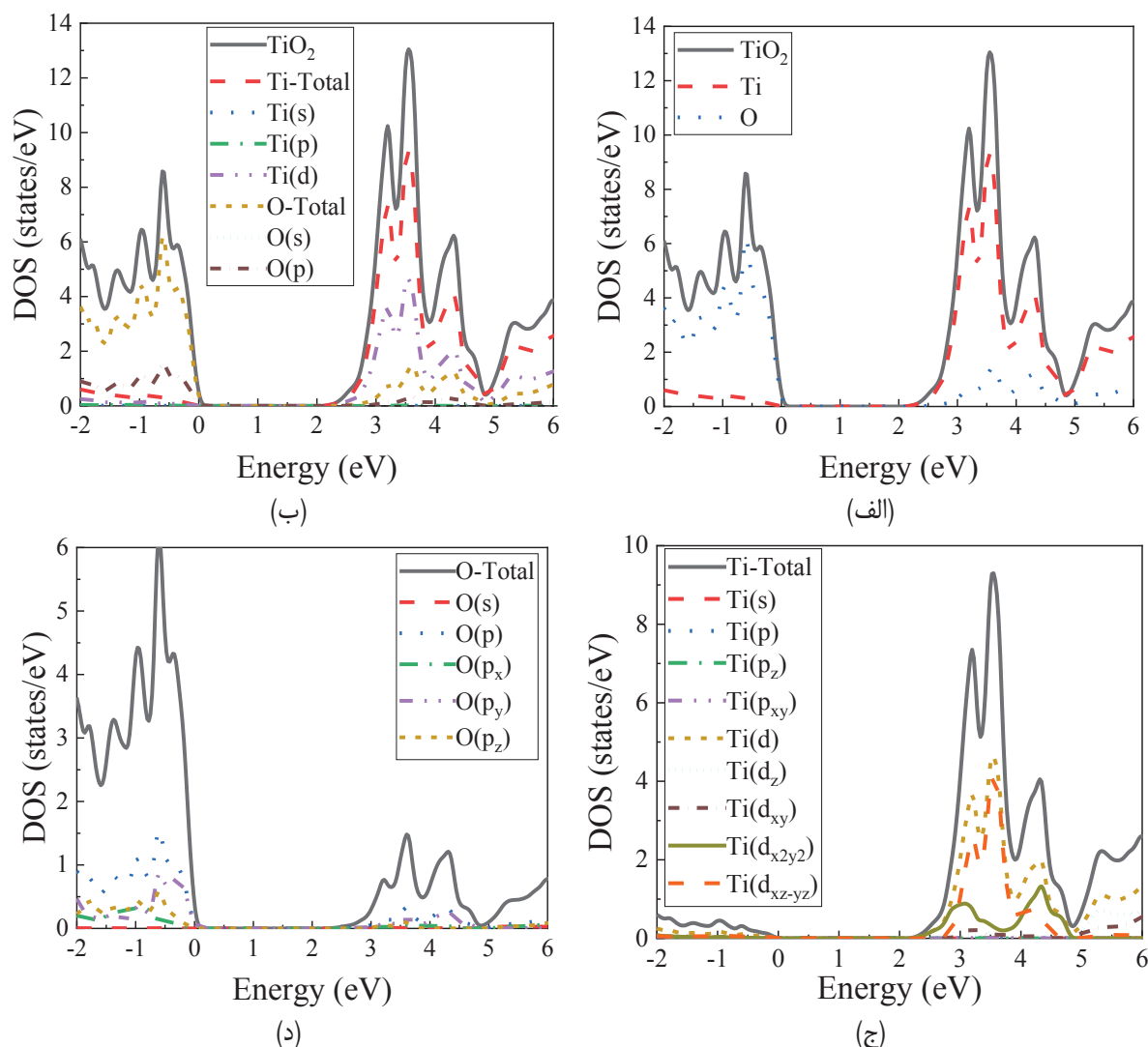
شکل ۵- نمودار الف) چگالی حالت‌های کل و ب) تا د) چگالی حالت‌های جزئی اتم‌های تشکیل‌دهنده ترکیب \text{TiO}_2
