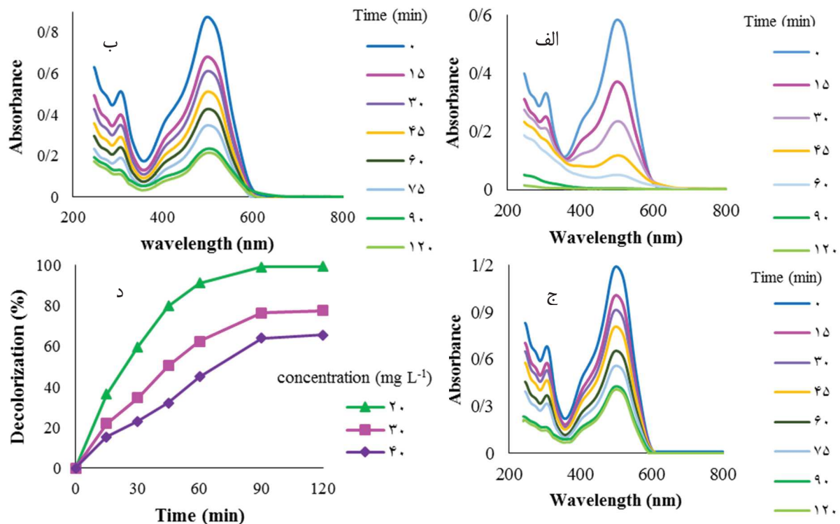
شکل ۱۳- رنگزدایی غلظت‌های مختلف رنگزای مستقیم قرمز ۲۳ توسط فوتوکاتالیست سنتز شده به روش احتراقی الف) بررسی اثر میزان غلظت بر رنگزدایی ( 20 \text{ mg L}^{-1} ب) ( 30 \text{ mg L}^{-1} ج) ( 40 \text{ mg L}^{-1} د)
