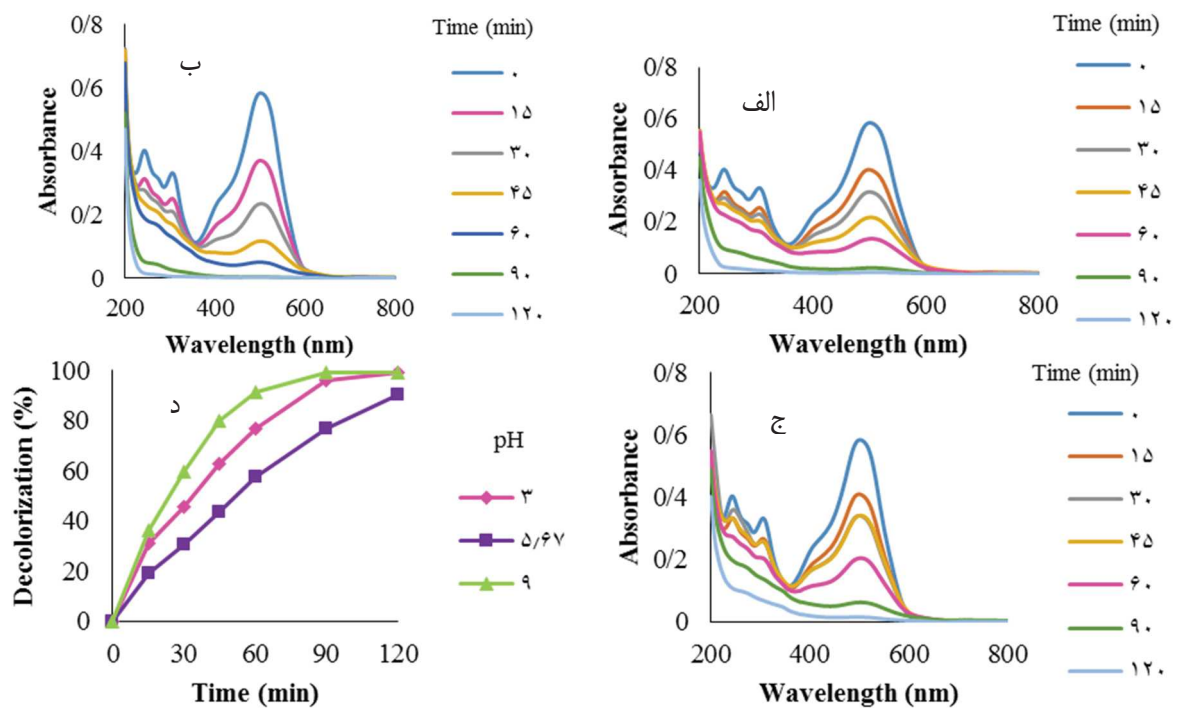
شکل ۱۲- رنگزدایی رنگزای مستقیم قرمز ۲۳ توسط فوتوکاتالیست سنتز شده به روش احتراقی با مقادیر مختلف pH (الف) (ب) (ج) 5/6.7 (د) بررسی اثر مقدار pH بر رنگزدایی
