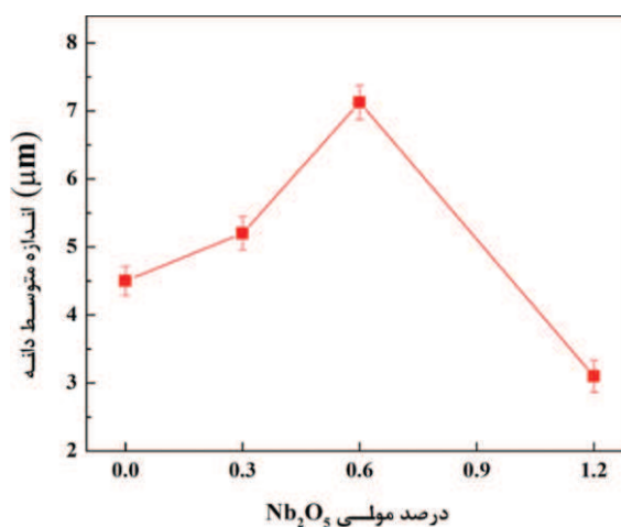
شکل ۴- تغییرات اندازه متوسط دانه نمونه‌ها بر حسب درصد مولی Nb 2 O 5 .
