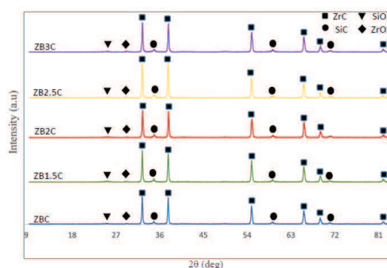
شکل ۳- الگوی پراش اشعه ایکس نمونه‌های سنتز شده با نسبت استوکیومتری تا ۳ برابر مول B 2 O 3
