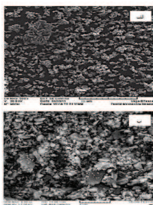
شکل ۶- تصویر SEM از پودر سیلیکات زیرکونیوم (الف) قبل از آسیاب و (ب) بعد از آسیاب
