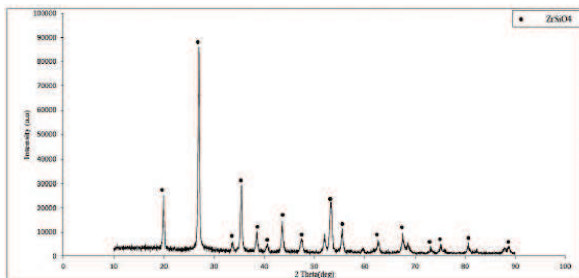
شکل ۱- الگوی XRD پودر سیلیکات زیرکونیوم
