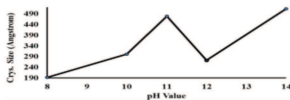
شکل ۵- نمودار قطر کریستالیت‌های نمونه‌های سنتز شده در دمای 750^{\circ}\text{C} به مدت ۲ ساعت
