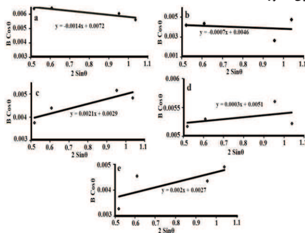
شکل ۴- نمودار ویلیامسون- هال نمونه‌های سنتز شده در دمای 750^{\circ}\text{C} به مدت ۲ ساعت؛ S8 (a)، S10 (b)، S11 (c)، S12 (d)، S14 (e)
