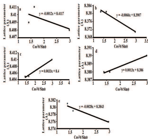
شکل ۶- نمودار توابع برون‌یابی برای نمونه‌های سنتز شده در دمای 750^{\circ}\text{C} به مدت ۲ ساعت؛ S8 (a)، S10 (b)، S11 (c)، S12 (d)، S14 (e)
