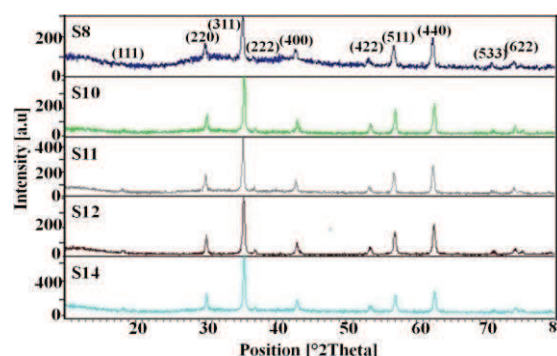
شکل ۲- تصویر XRD پودرهای سنتزی در شرایط pH مختلف در دمای 750^\circ\text{C} به مدت ۲ ساعت
