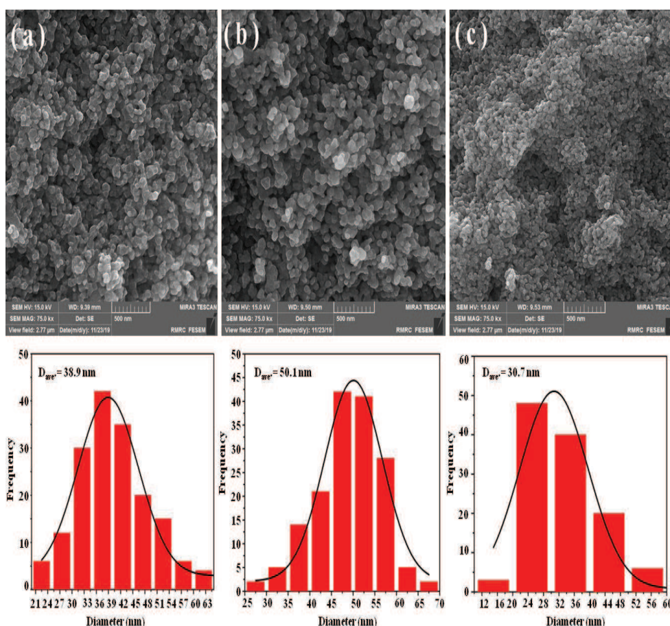
شکل ۸- میکروگراف نمونه‌های سنتز شده در دمای 750^{\circ}\text{C} به مدت ۲ ساعت: S8 (a) و S11 (b) و S14 (c).
