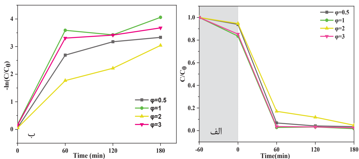
شکل ۶- الف) نمودار تخریب فوتوکاتالیستی ب) نمودار سرعت واکنش رنگدانه‌ی MB تحت نور فرابنفش اکسید روی سنتز شده در نسبت‌های سوخت به اکسندۀ متفاوت.
