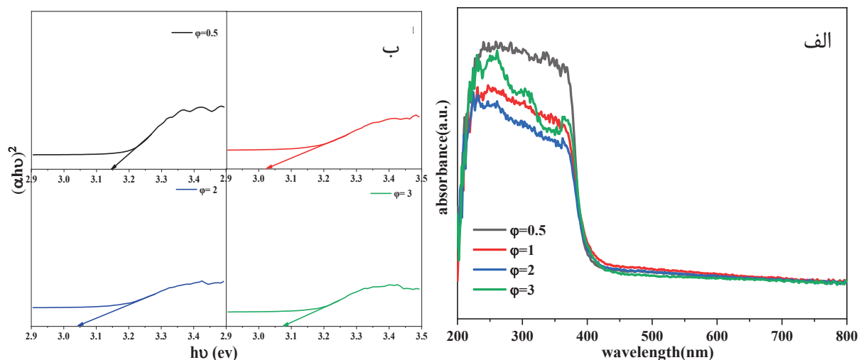
شکل ۵- الف) طیف جذبی ب) نمودار (\alpha h\nu)^2 بر حسب انرژی فوتون اکسید روی سنتز شده با نسبت‌های متفاوت
